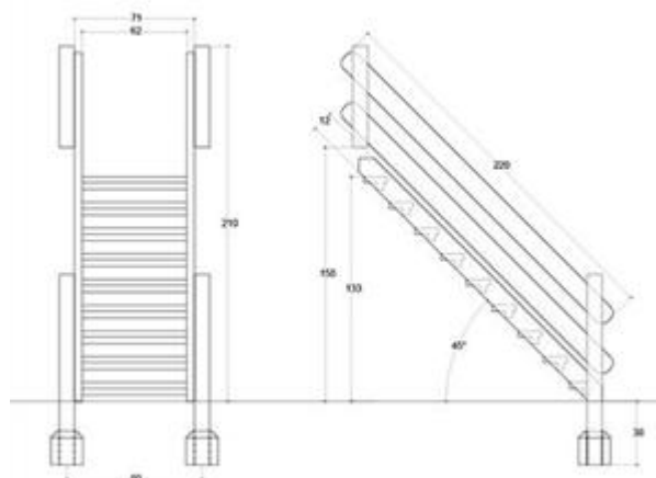
SCALA PER PEDANA H 150 CM
