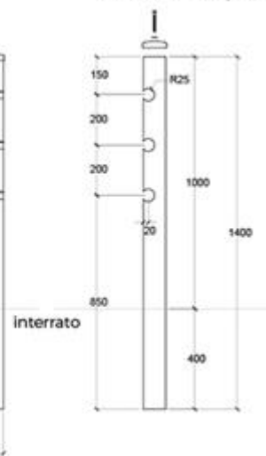
vista laterale / esploso
