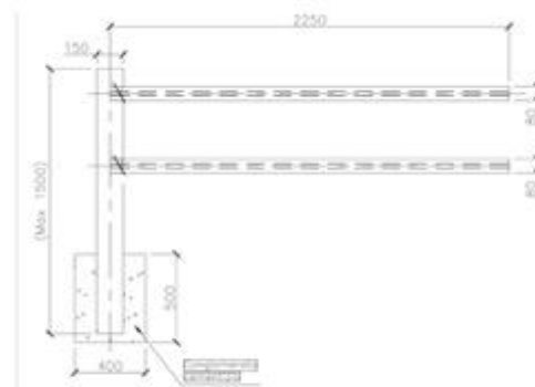
Versione con interasse 225 cm
