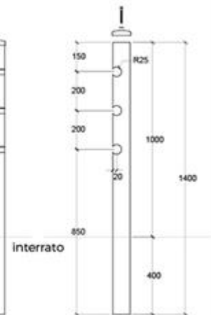
vista laterale / esploso
