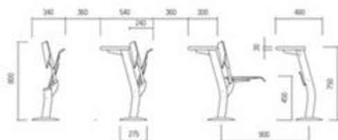
banco con piano fisso
