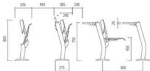
banco con piano fisso
