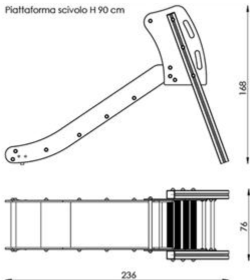
Piattaforma scivolo H 90 cm
